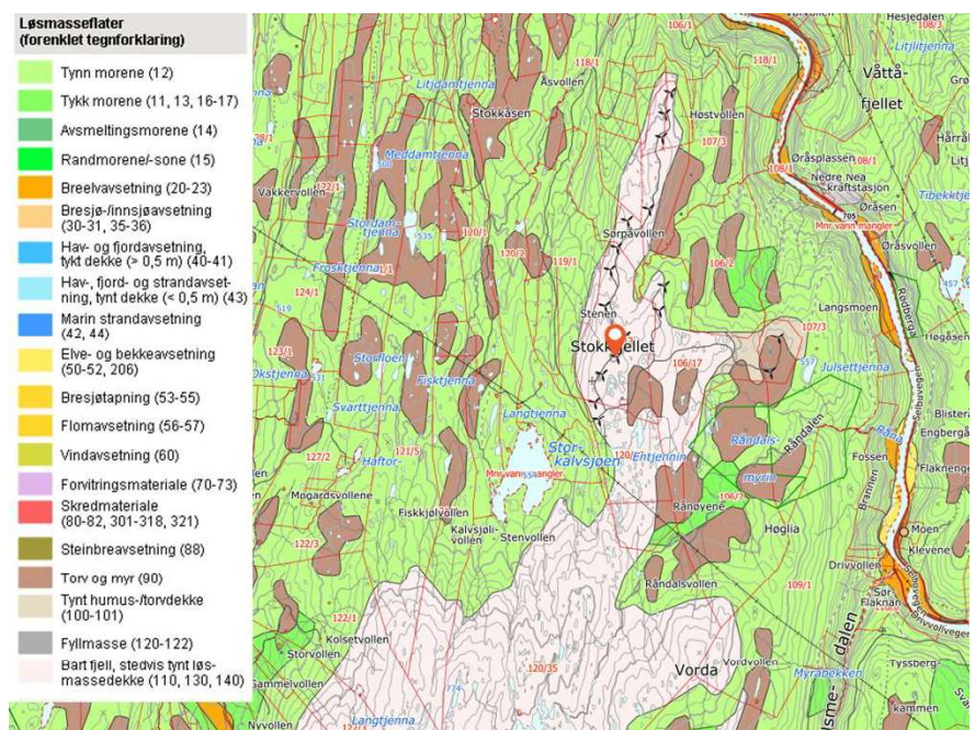
Figur 11 Bart fjell og områder med torv og myr er løsmassene som er vist ved Stokkfjellet vindkraftverk i NGUs løsmassekart. Adkomstvegen ligger innenfor et område vist med morenemasser. Kilde: NGU kart
