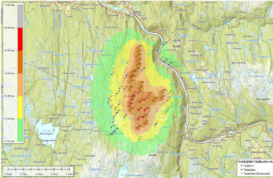
Figur 24 Støysonekart basert på beregnet støynivå for verste scenario (medvind fra alle retninger).
